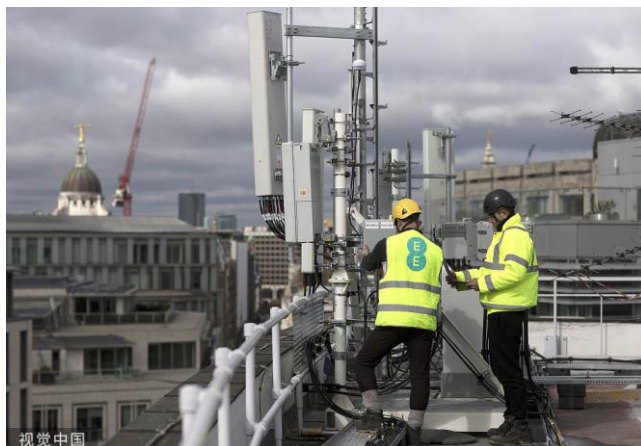
当地时间 2019 年 3 月 15 日，英国伦敦，英国移动运营商 EE 的工程师在检查华为公司的 5G 相关设备。
